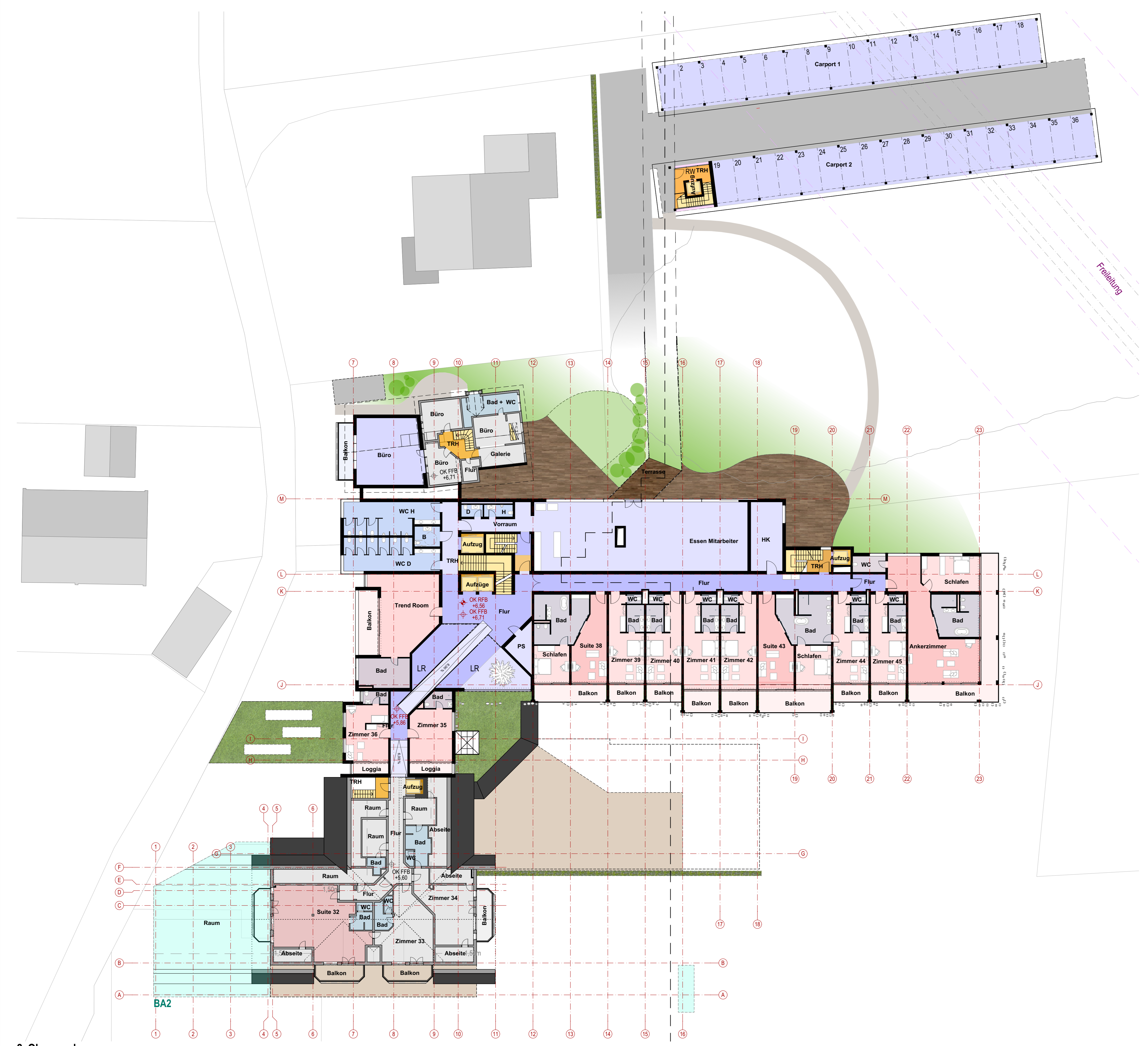
2. Obergeschoss
