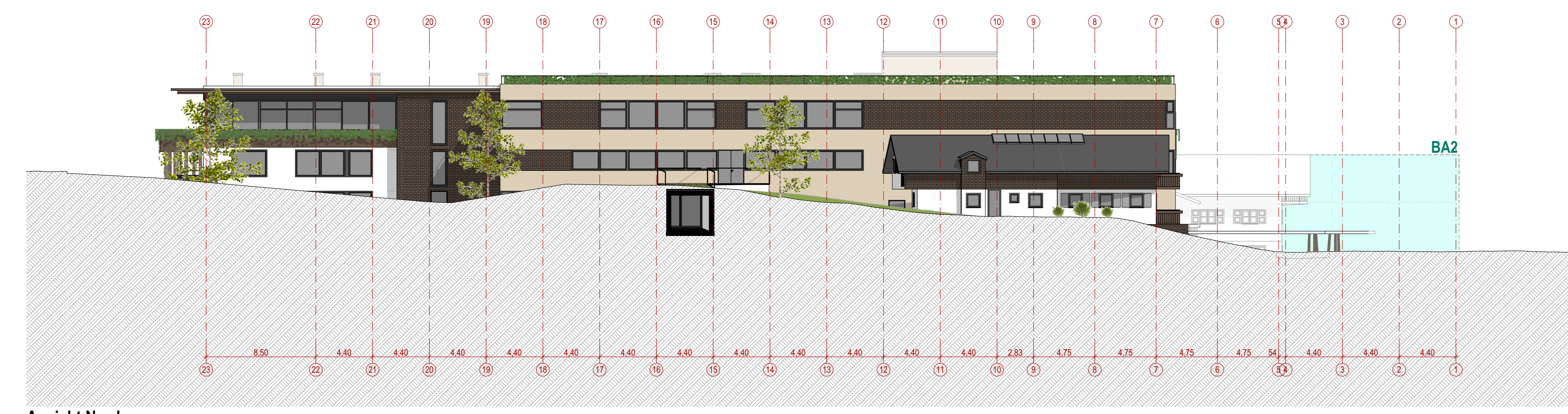
Ansicht Nord
